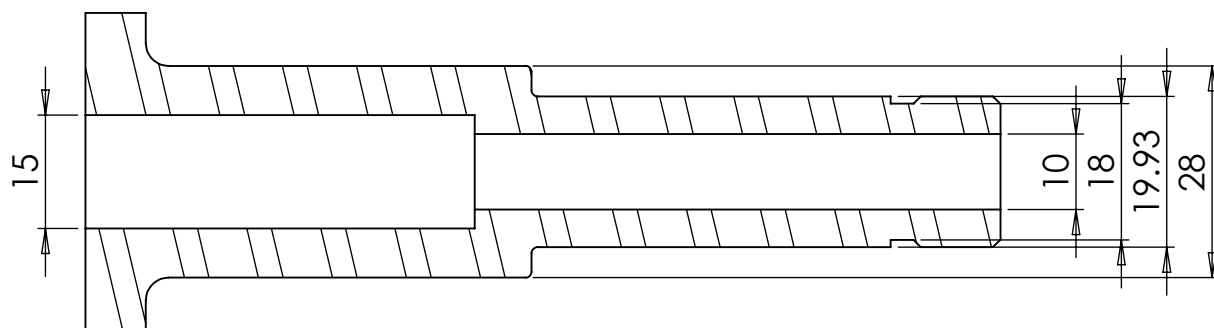
SEZIONE A-A SCALA 1:1
